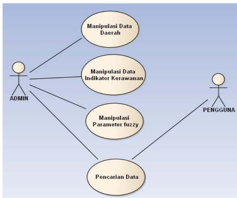
Gambar 3. Use Case Sistem Fuzzy Identifikasi Daerah Rawan Pangan
