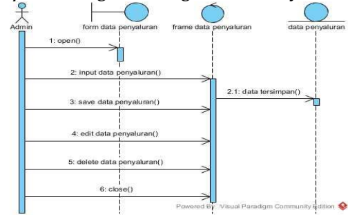
Sumber : Hasil Penelitian (2018) Gambar 8. Sequence Diagram Mengisi Data Penyaluran
