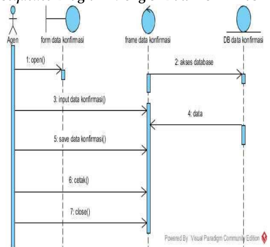
Gambar 13. Sequence Diagram Mengisi Data Konfirmasi
