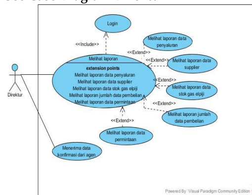
Sumber : Hasil Penelitian (2018) Gambar 3. Use Case Diagram Direktur
