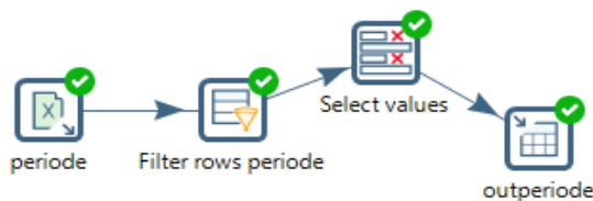
Gambar 7. ETL dim_periode
