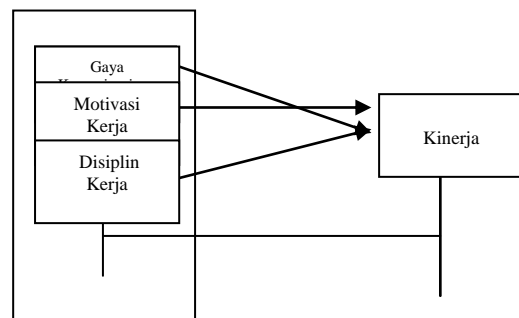
Gambar 2.1 Kerangka Pemikiran
