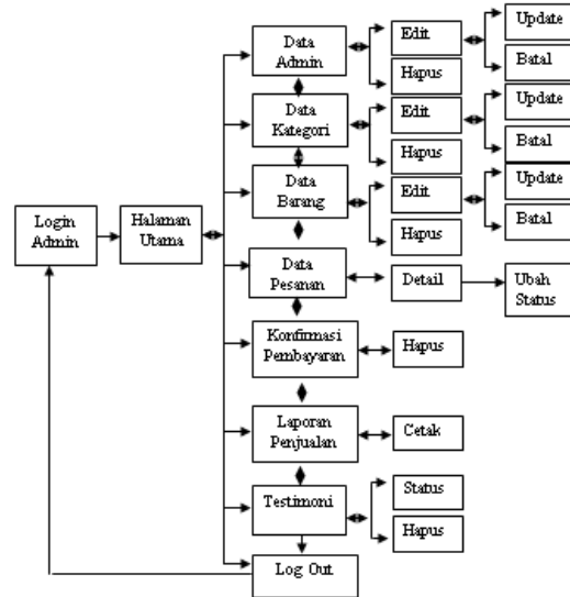
Gambar 6. Struktur Navigasi Halaman Admin Sumber: Hasil penelitian (2014)
