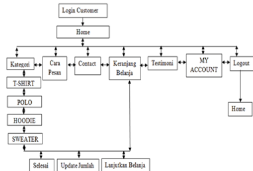
Gambar 7. Struktur Navigasi Halaman Customer Sumber: Hasil penelitian (2014)
