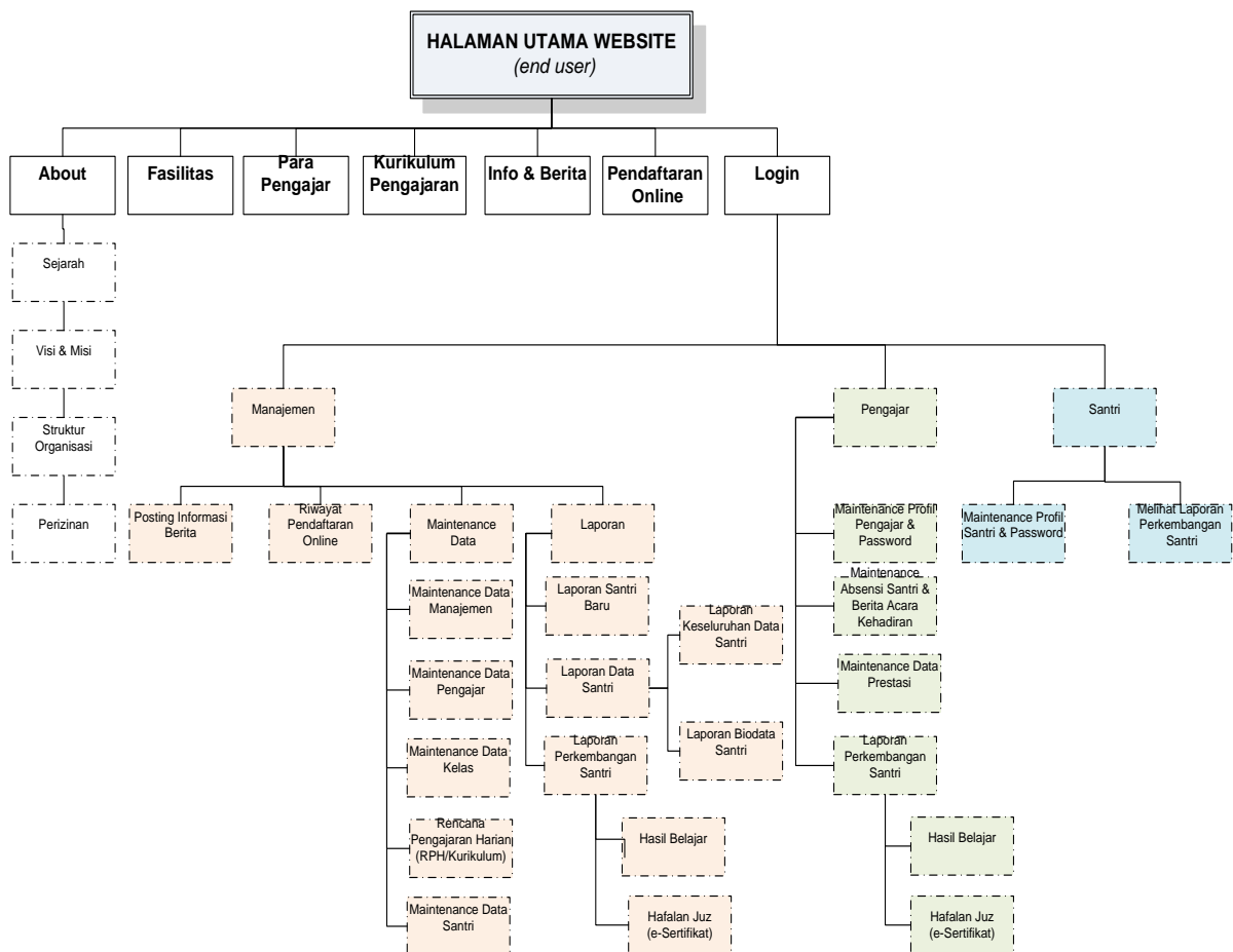
Gambar 1 Struktur Navigasi Website Rumah Tahfidz dan TPQ Sakinah
