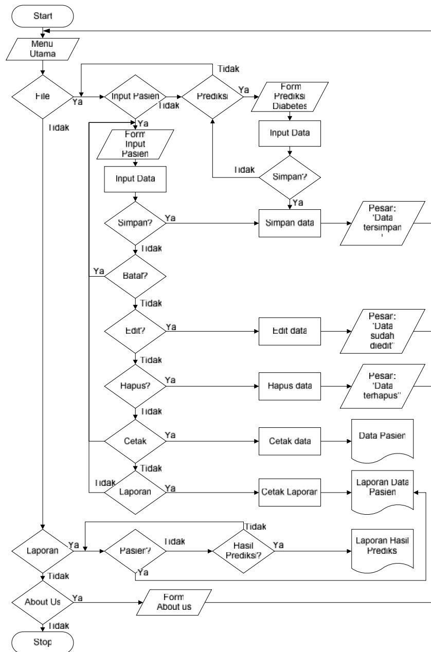
Gambar 6. Flowchart Sistem Prediksi Penyakit Diabetes
